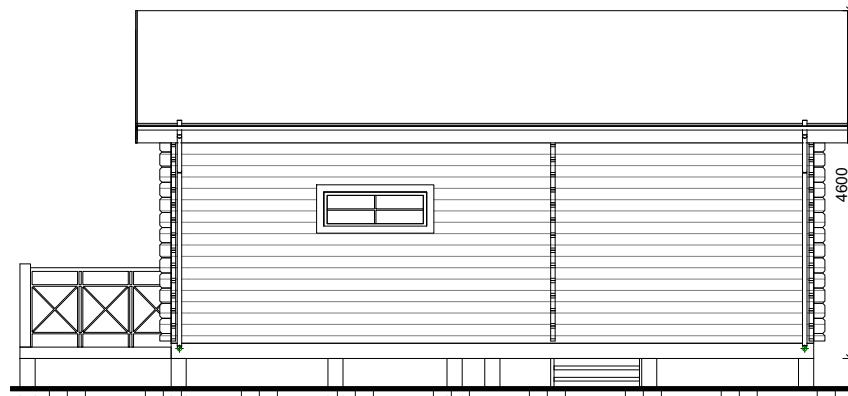
3 Fasad 1 1 : 100
