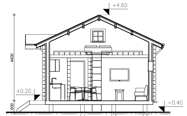
2 Sektion 1 1 : 100
