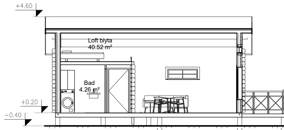
1 Sektion 2 1 : 100
