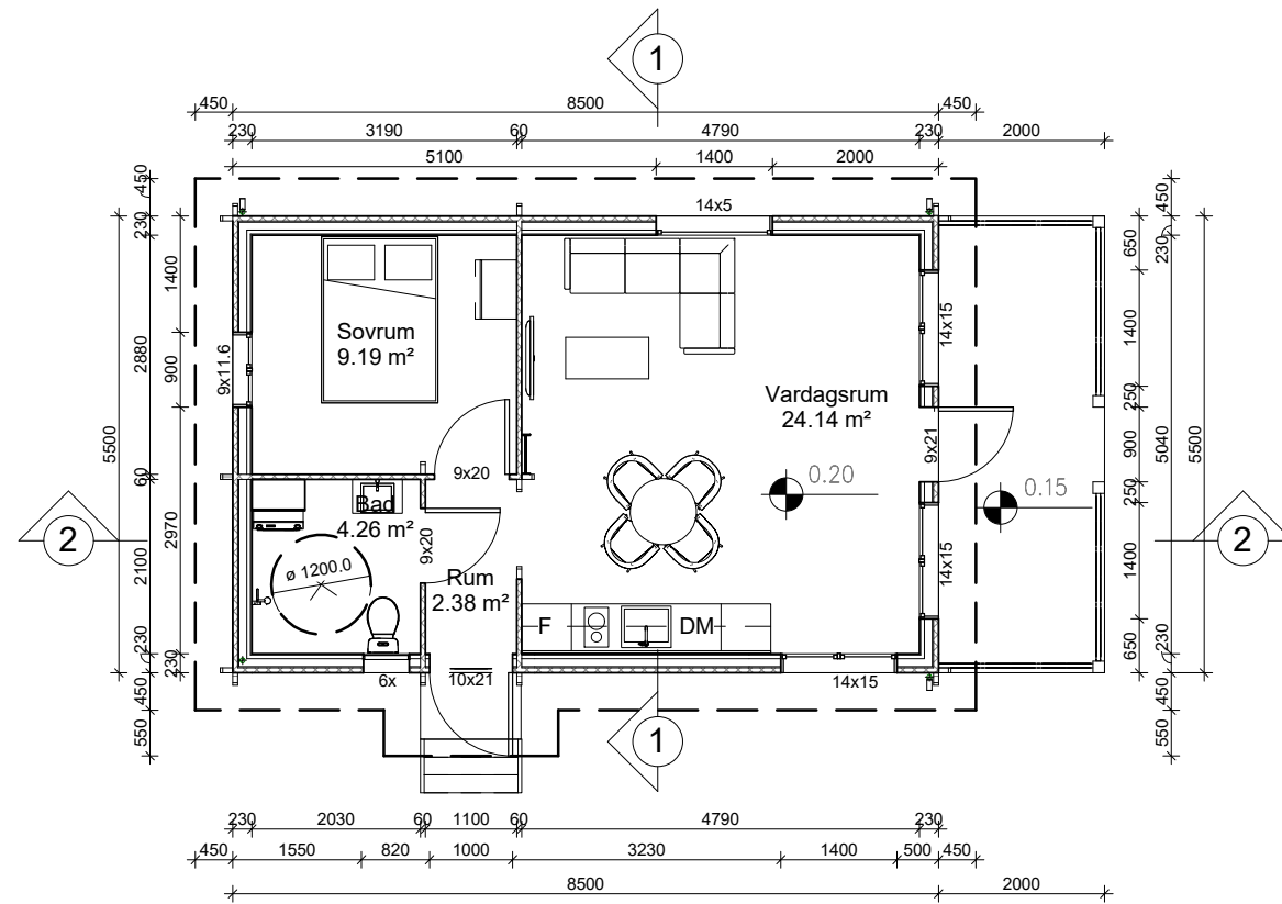
1 Marknivå 1 : 100
