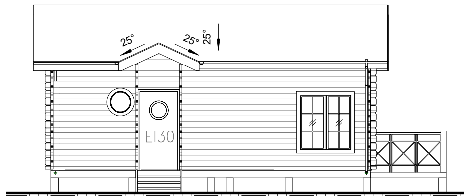
5 Fasad 2 1 : 100
