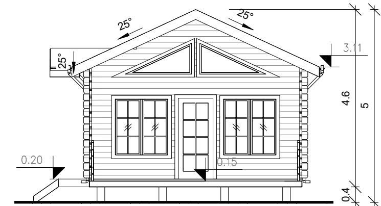
4 Fasad 4 1 : 100
